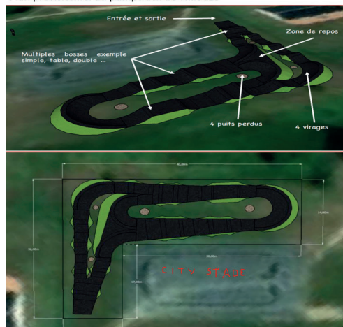
Plan prévisionnel du pumptrack de Thilouze
